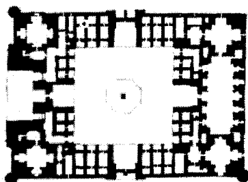
FIGURA 6. Plano de la madrasa Ulug Beg.
